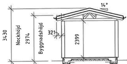
Öppen kort takfot SEKTION
